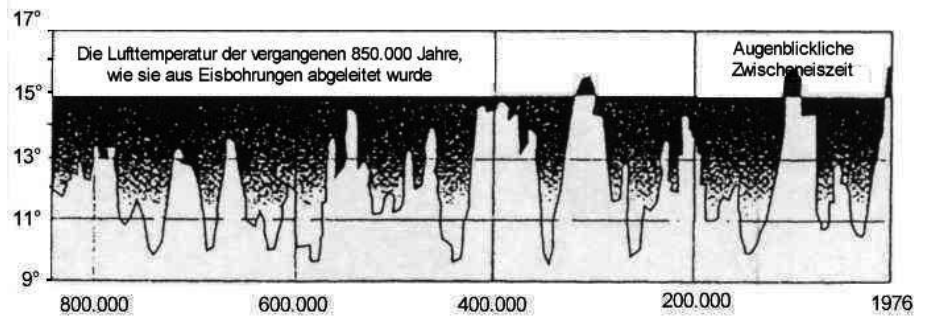
Abb. 8: In den letzten 800.000 Jahren gab es ein ständiges Auf und Ab der Erdtemperaturen mit Schwankungen zwischen +10 und +16^{\circ}\text{C} (Meier, „Die Mär von der Klimakatastrophe“).
