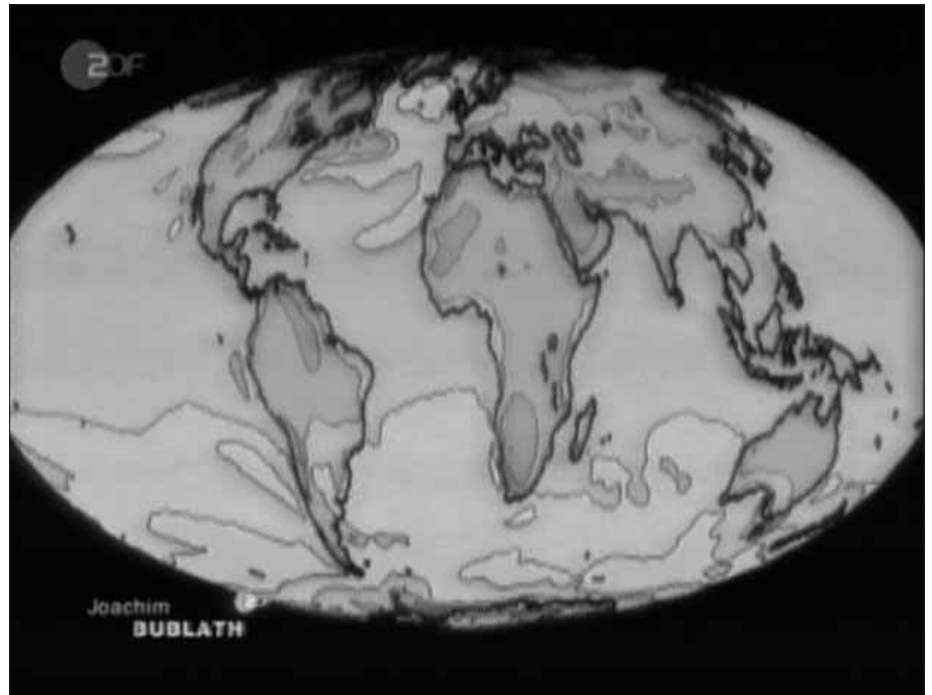
Abb. 13: Per Computer-Hochrechnung erstelltes Wärmebild der Erde der Zukunft (Bublath, ZDF)
