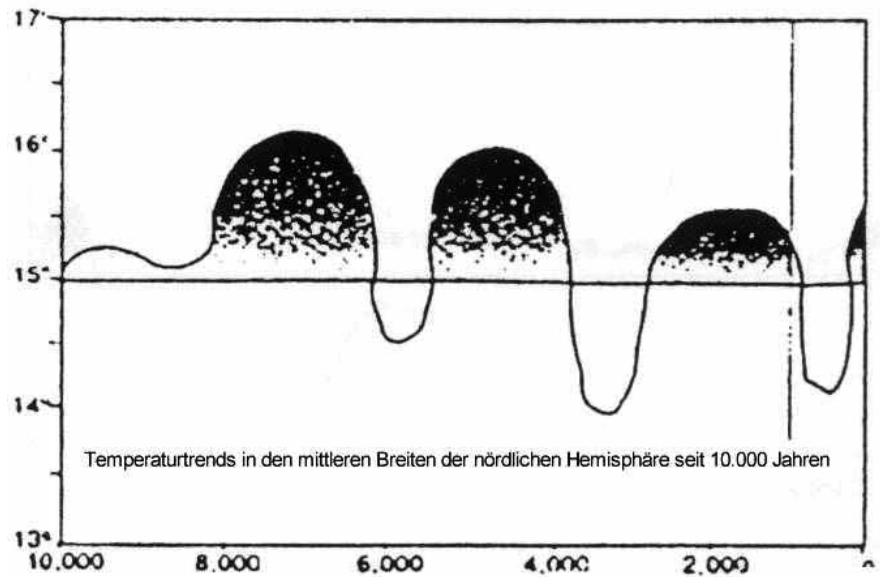
Abb. 9: In den vergangenen 10.000 Jahren gab es mindestens drei Kälte- und vier Wärmeperioden (Meier, „Die Mär von der Klimakatastrophe“)
