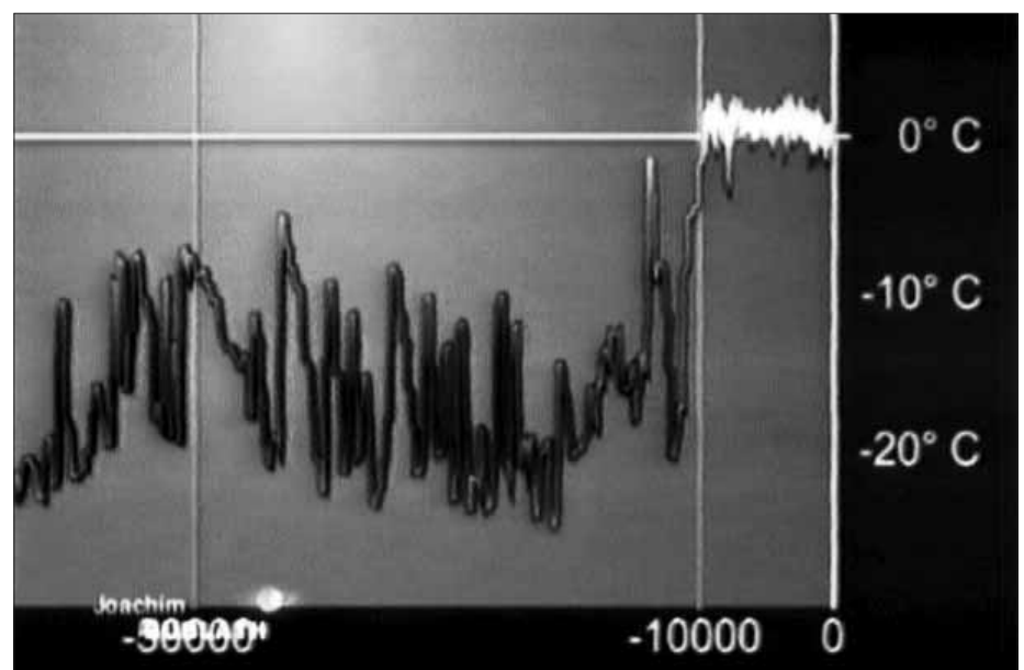
Abb. 3: Temperatur-Entwicklung der Erde in den letzten 50.000 Jahren (Bublatz, ZDF)
