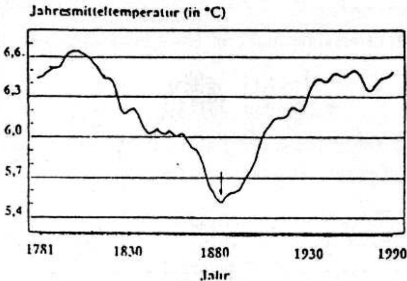
Abb. 5: Die Entwicklung der Jahresmitteltemperaturen von 1781 bis 1990 auf der Station Hohenpeissenberg (Meier, „Die Mär von der Klimakatastrophe“).
