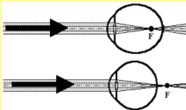
Oben: Kurzsichtiges Auge. Der Brennpunkt (F) des scharfen Bildes liegt vor der Netzhaut im Glaskörper. Unten: Weitsichtiges Auge. Der Brennpunkt (F) liegt hinter der Netzhaut. Beide Bilder erscheinen unscharf.
